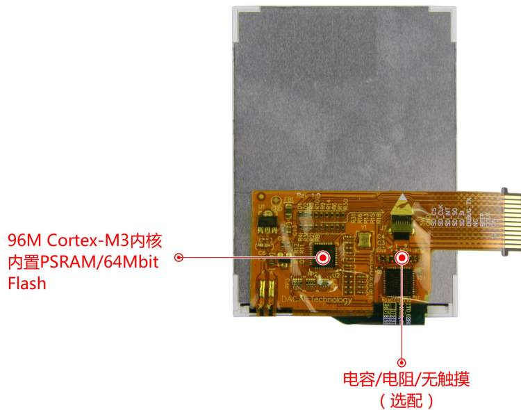
图 1-4 硬件配置图
