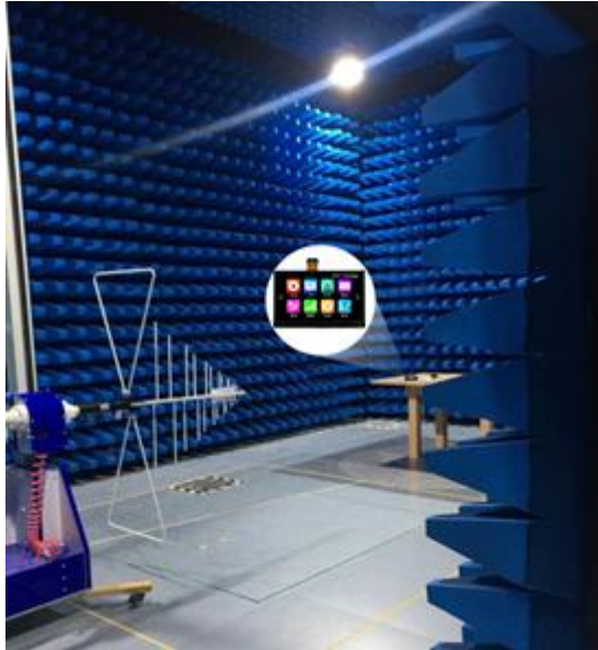
图 7-5 辐射测试图
