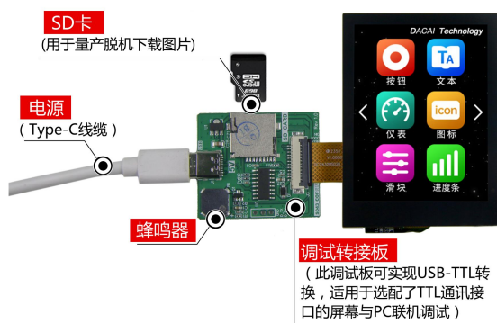
图 1-5 调试工具图
